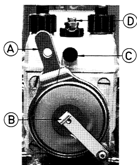
Bild 17 Tändapparat för 0-11 och 0-21
