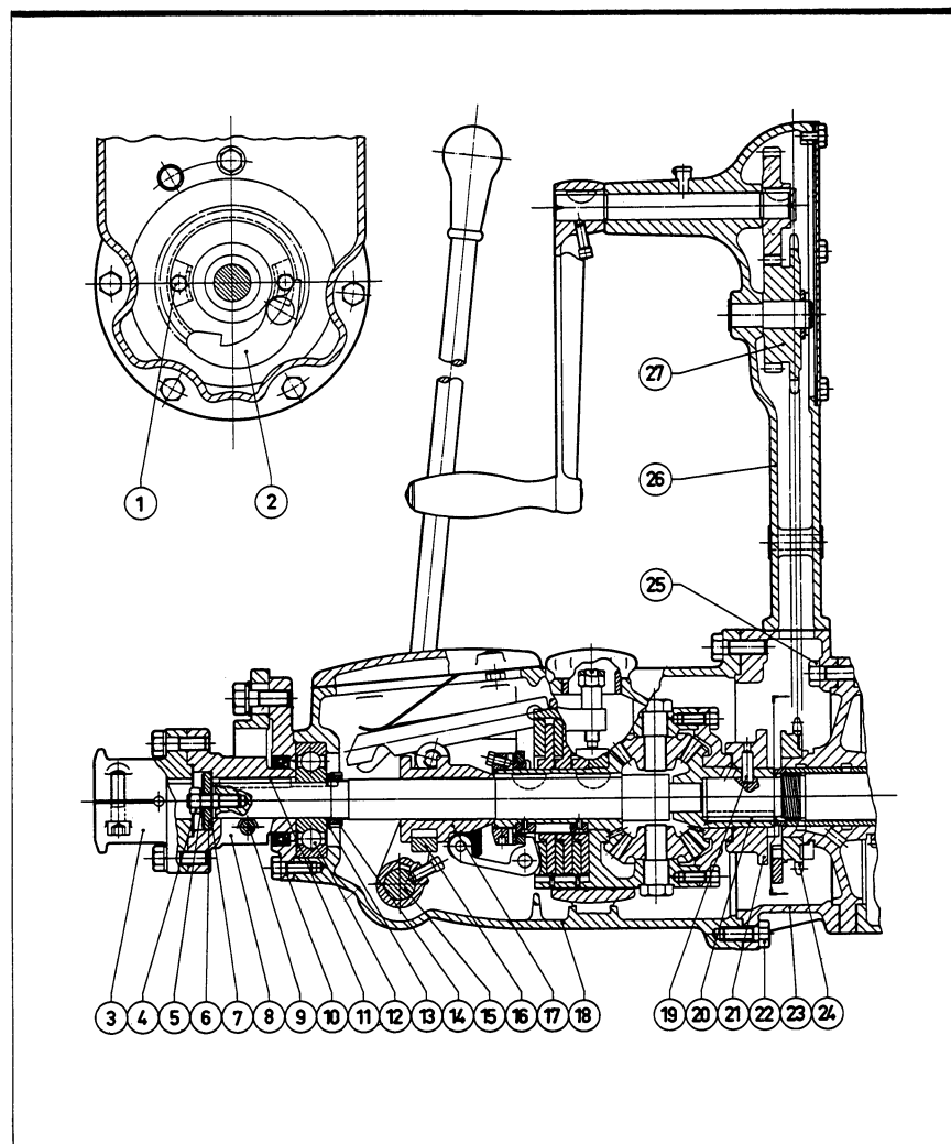
Bild 2 Backslag och kedjestart i genomskäring
